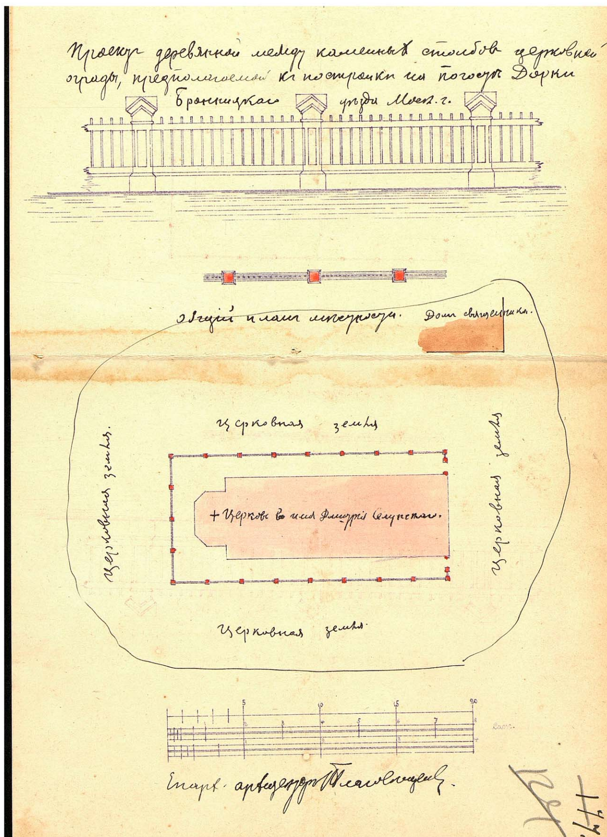
6. Проект предполагаемой ограды церкви Дмитрия Солунского, что в Дорках. Общий план местности. 1901 г. ЦХД до 1917 г. Ф. 54. Оп. 155. Д. 15. Л. 124.
